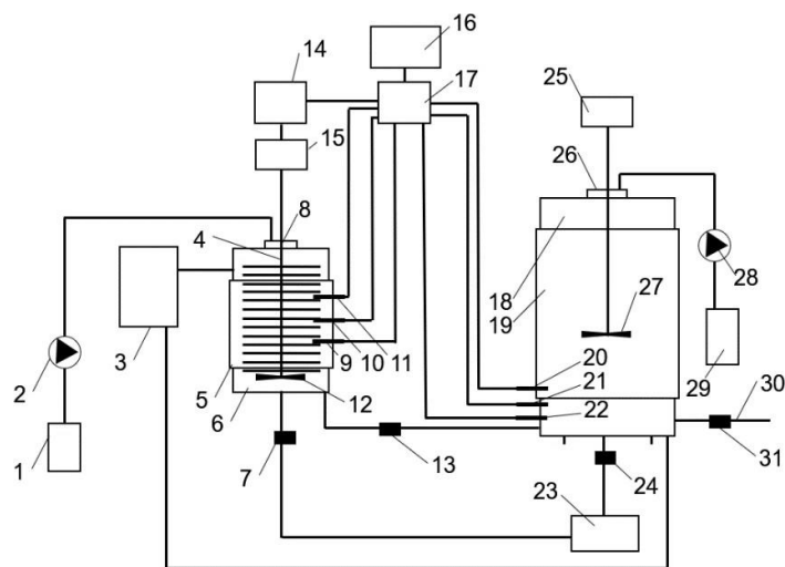
Рисунок 10 – Блок-схема биореактора
