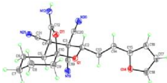
Рис. 6 Молекула соединения 6в
