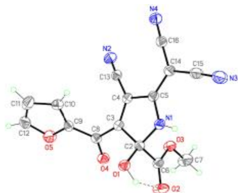
Рис. 4 Молекула соединения 56
