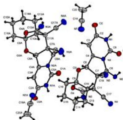
Рис. 8 Молекула соединения 7
