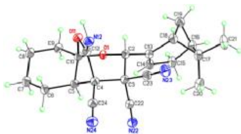
Рис. 7 Молекула соединения 6з
