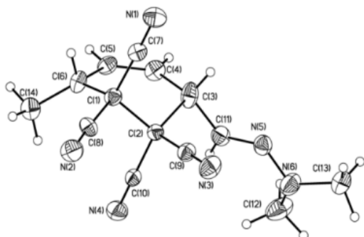
Рис. 3 Молекула соединения 4a
