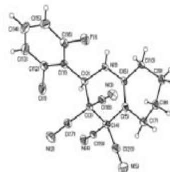
Рис. 9 Молекула соединения 8в
