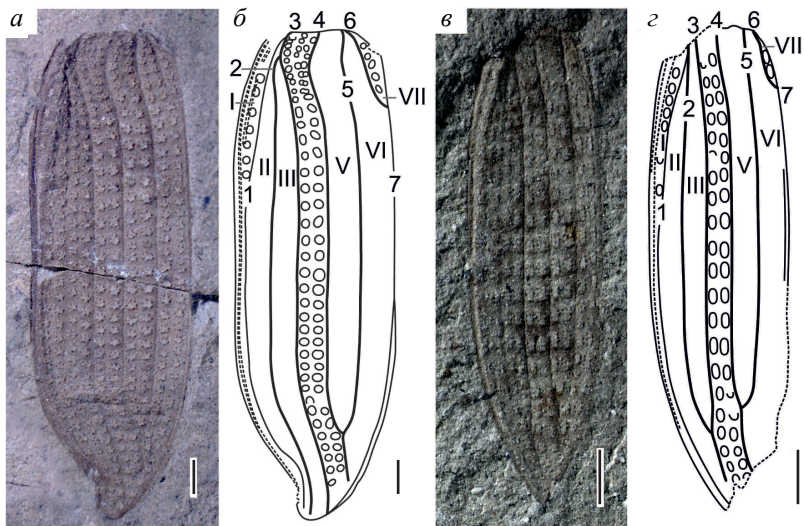
Рис. 4. Варианты жилкования надкрылий исследованной группы жуков. а-б – Z. alexrasnitsyni : а – фото, б – рисунок; в-г – N. elegans : в – фото, г – рисунок. Римскими цифрами подписаны поля, арабскими – жилки. Длина масштабной линейки 1 мм.
