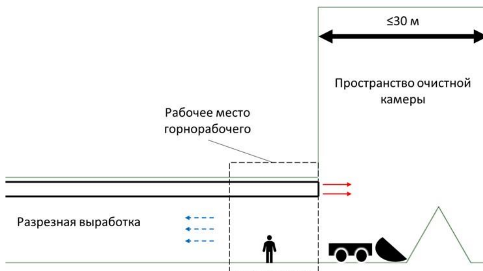
Рисунок 1 – Тупиковая очистная камерообразная горная выработка, образующаяся за счет расширения разрезной выработки, с указанием рабочего места горнорабочего
