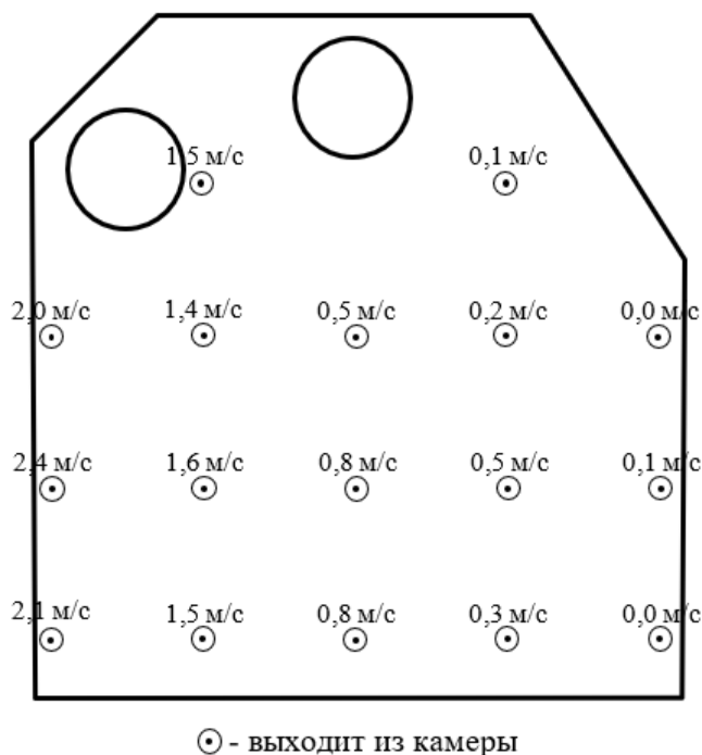
Рисунок 2 – Результаты измерения поля скоростей движения воздуха в исследуемом сечении разрезной выработки КАМ-11-15-на_3 подземного рудника «Маяк»
