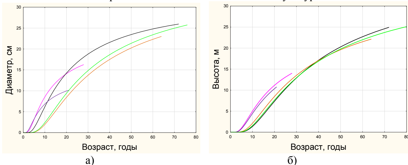
Рисунок 2 – Ход роста по диаметру (а) и высоте (б) лесных культур на ограниченно лесопригодных и условно лесопригодных почвах — ПП-89, — ПП-84, — ПП-88, — ПП-96, — ПП-69
