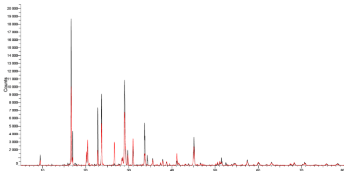
Рисунок 4 – Результаты рентгенофазового анализа огнетушащего порошка «Волгалит-ABC» (черный) и огнетушащего порошка «Волгалит-ABC» с гидрофобно-модифицирующей добавкой марки «ГМД-20NT» (красный)
