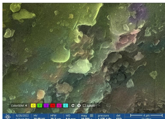
Рисунок 5 – Результаты энергодисперсионной рентгеновской спектроскопии огнетушащего порошка «Волгалит-ABC» с гидрофобно-модифицирующей добавкой марки «ГМД-20NT»
