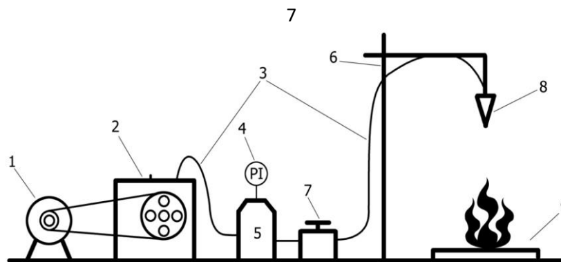
Рисунок 1 – Принципиальная схема лабораторной установки для исследования огнетушащей способности порошковых составов
