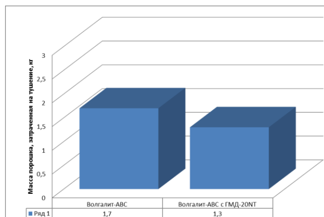
Рисунок 7 – Количество порошка, затраченное на тушение модельного очага пожара класса 55В огнетушащим порошком «Волгалит-ABC» с гидрофобизирующей добавкой ГМД-20NT (1,5 % по массе)
