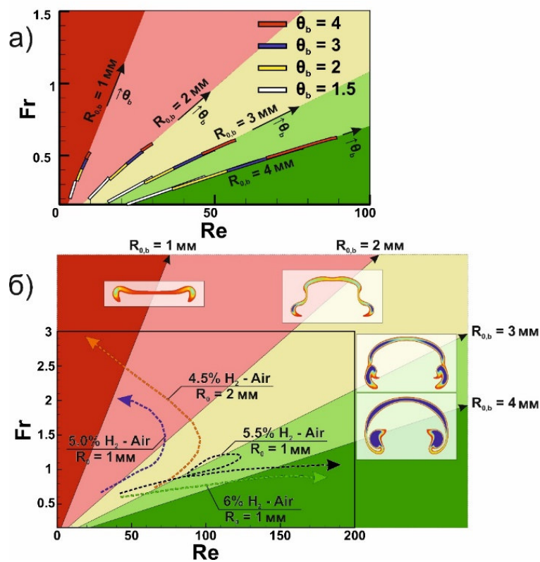
Рисунок 27. Диаграмма в координатах Re - Fr . а) Линейные сегменты соответствуют расчетам химически неактивных газовых пузырьков. Линейные аппроксимации этих
