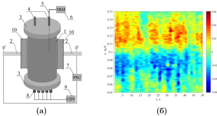
Рис. 2. (а) — схема эксперимента; (б) — пространственно-временная карта z -компоненты скорости течения вдоль оси цилиндра, сила тока I = 465 А
