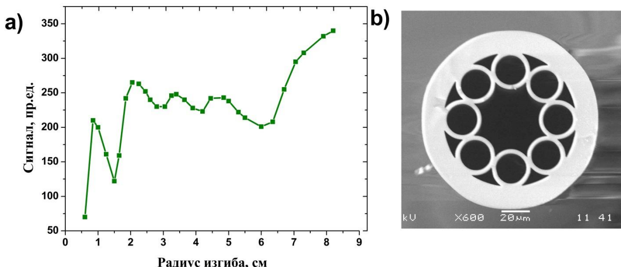
Рис. 6. (a) Зависимость интенсивности пропускаемого излучения от радиуса изгиба РС на длине волны 1,06 мкм; (b) СЭМ-фотография торца световода, использованного в эксперименте [3].
