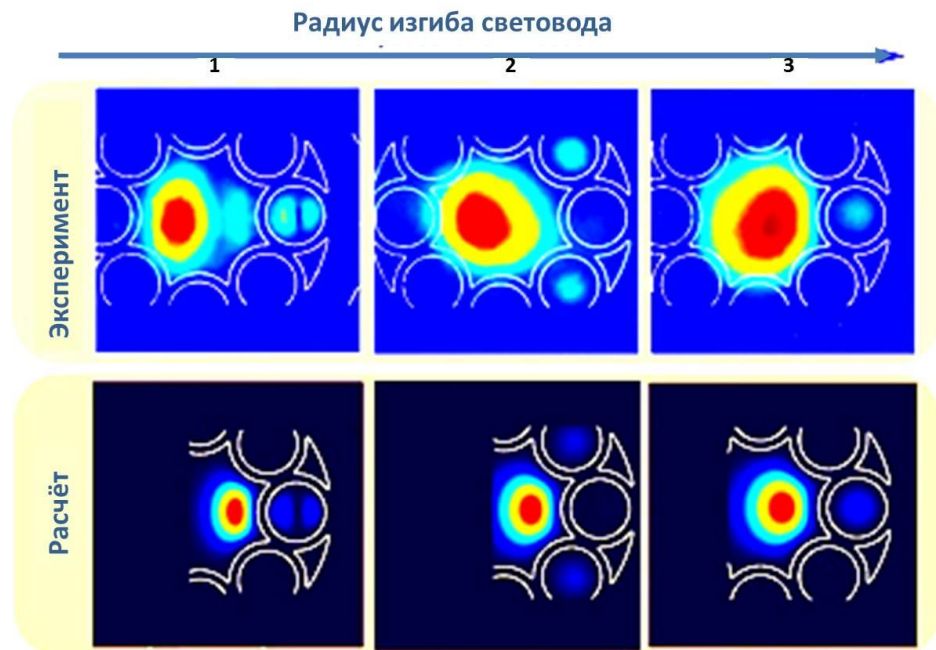
Рис.7. Измеренные экспериментально (вверху) и рассчитанные численно (внизу) распределения интенсивности излучения в ближнем поле на выходе изогнутого РС, соответствующие первым трём резонансным связям основной моды полой сердцевины с модами капилляров оболочки. Расчётное распределение поля для радиусов изгиба 1,6, 3,6 и 5,6 см представлены на кадрах 1, 2 и 3, соответственно. Длина волны излучения 1,06 мкм. Ось изгиба находится слева. Масштаб: ширина каждого кадра 93 мкм; на каждом кадре указано положение основных элементов конструкции РС [3].
